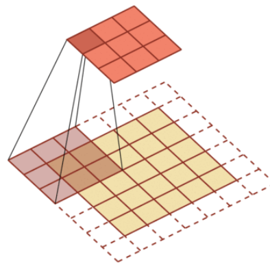
步长2, 零填充1
