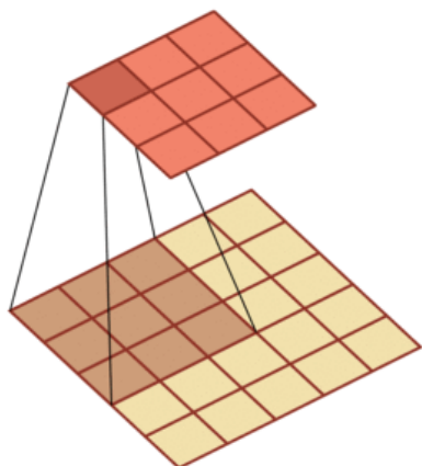
步长1, 零填充0
