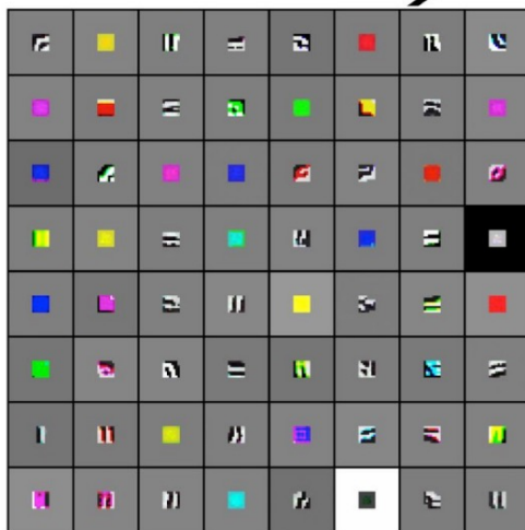
VGG-16 Conv1_1
